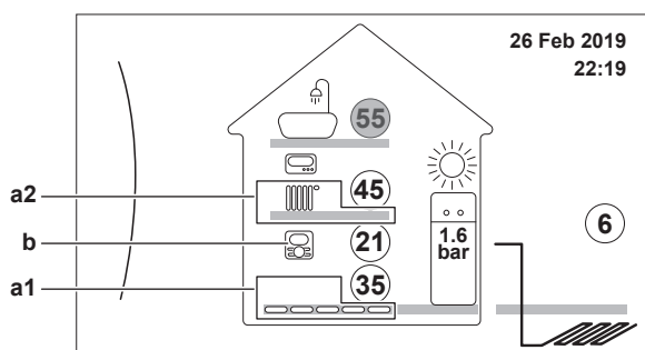
a1 Grelno telo v glavnem območju (v tem primeru Talno ogrevanje)
