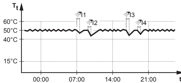
T_t Temperatura do depósito de AQS t Hora
