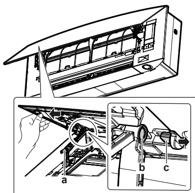
a Ručica b Prorez za osovinu c Osovina
