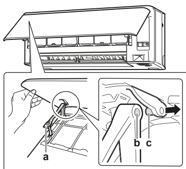
a Braç b Ranura del pivot c Pivot
