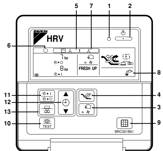
BRC301B61: Dálkový ovladač jednotky VRV
