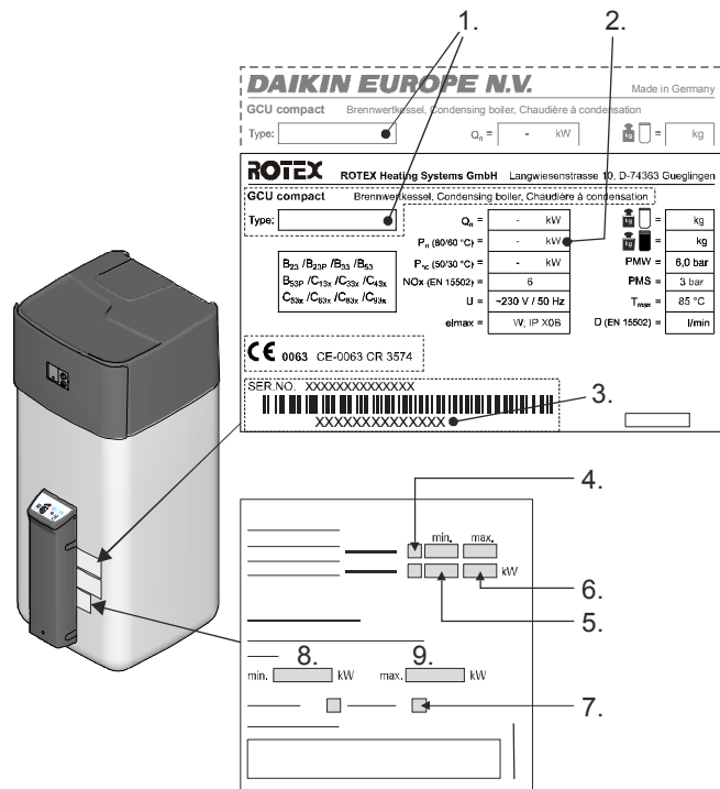
Afb. 1-1 Typeplaatje (boven) en Instellingssticker (onder)
