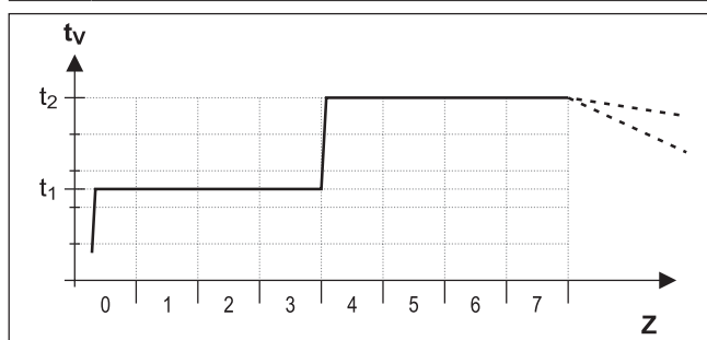
Bild 4-5 Zeitlicher Ablauf des Estrichprogramms beim Funktionsheizen
