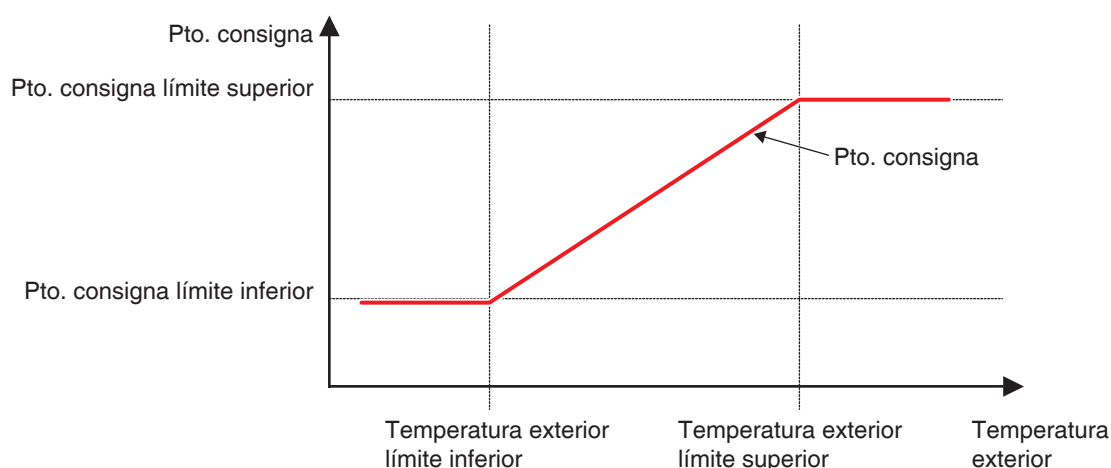
Relación entre la temperatura exterior y el pto. consigna
