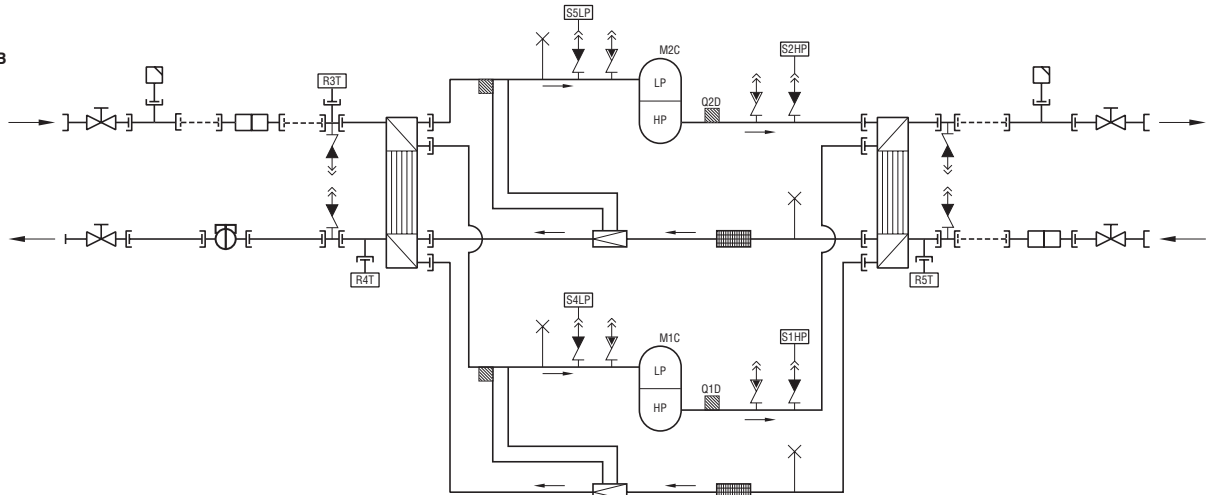
Abbildung – Funktionsplan
