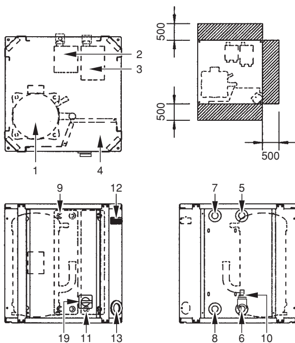
Slika - Glavni sestavni deli
