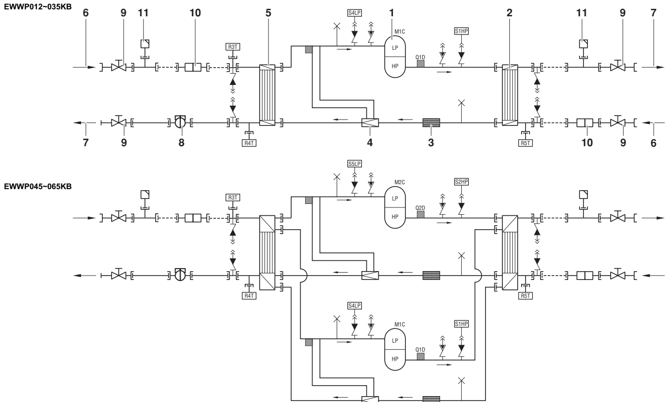
Slika - Shema funkcionalnosti
