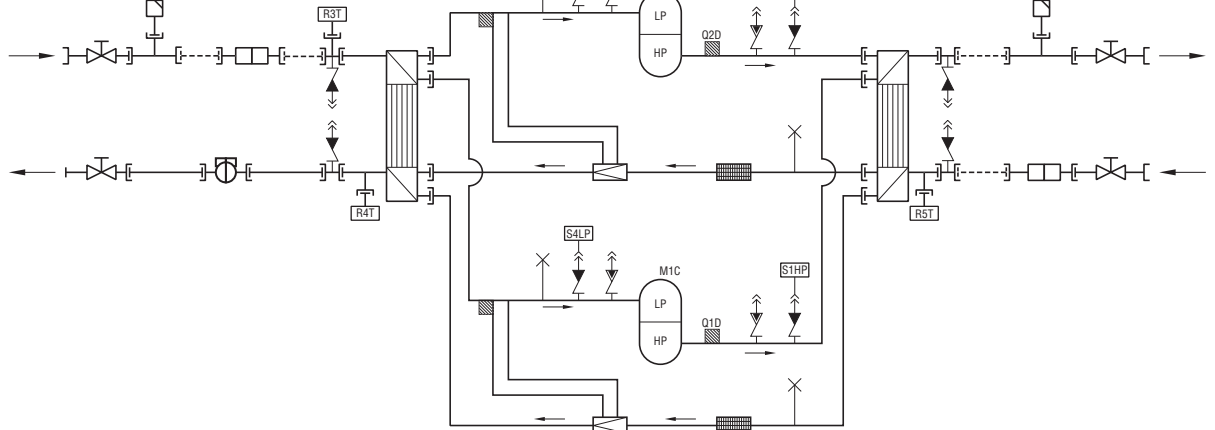
Рисунок: Функциональная схема чиллера
