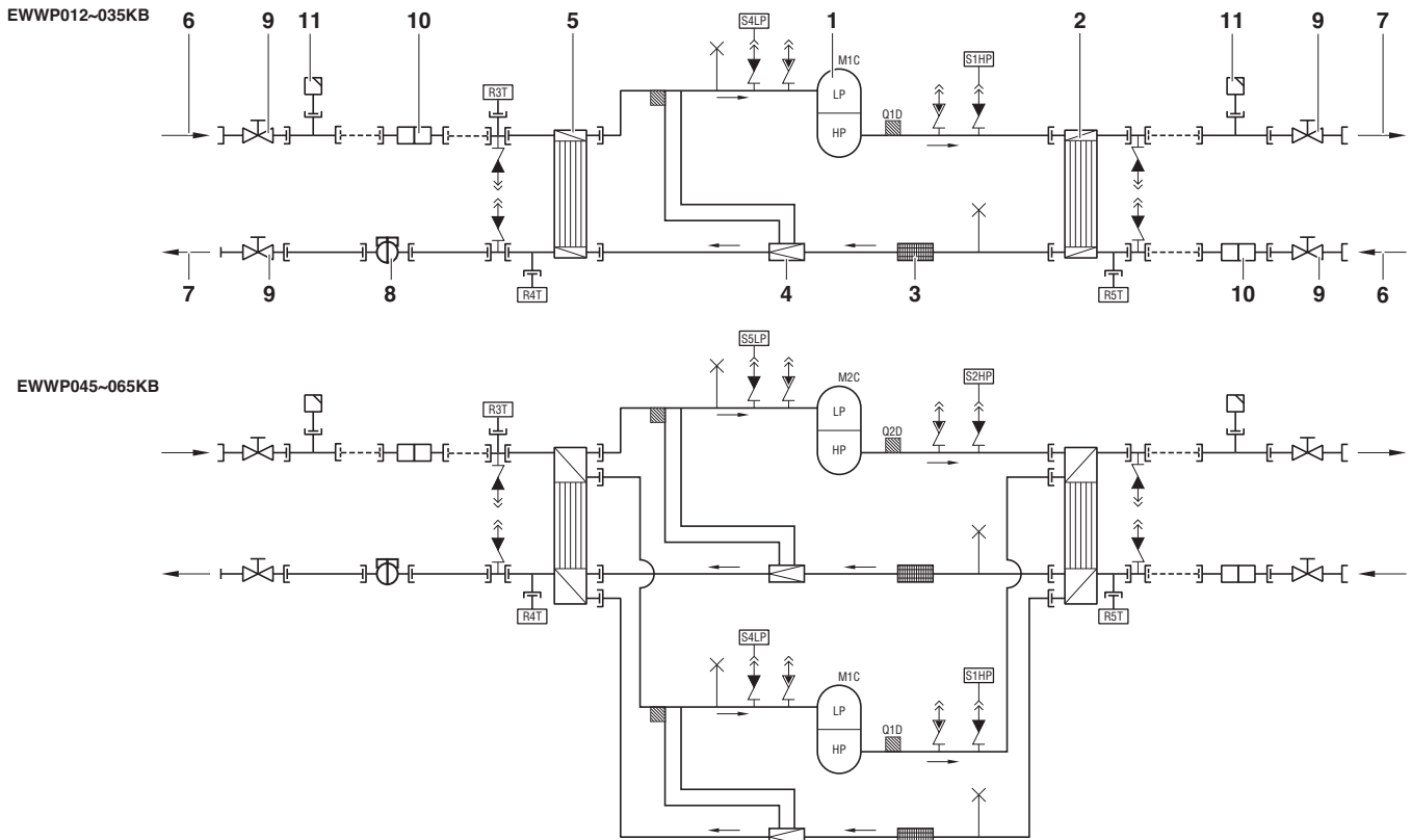
Abbildung – Funktionsplan
