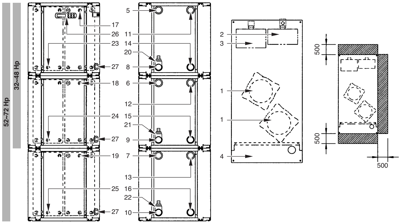
Figur - Hovedkomponenter
