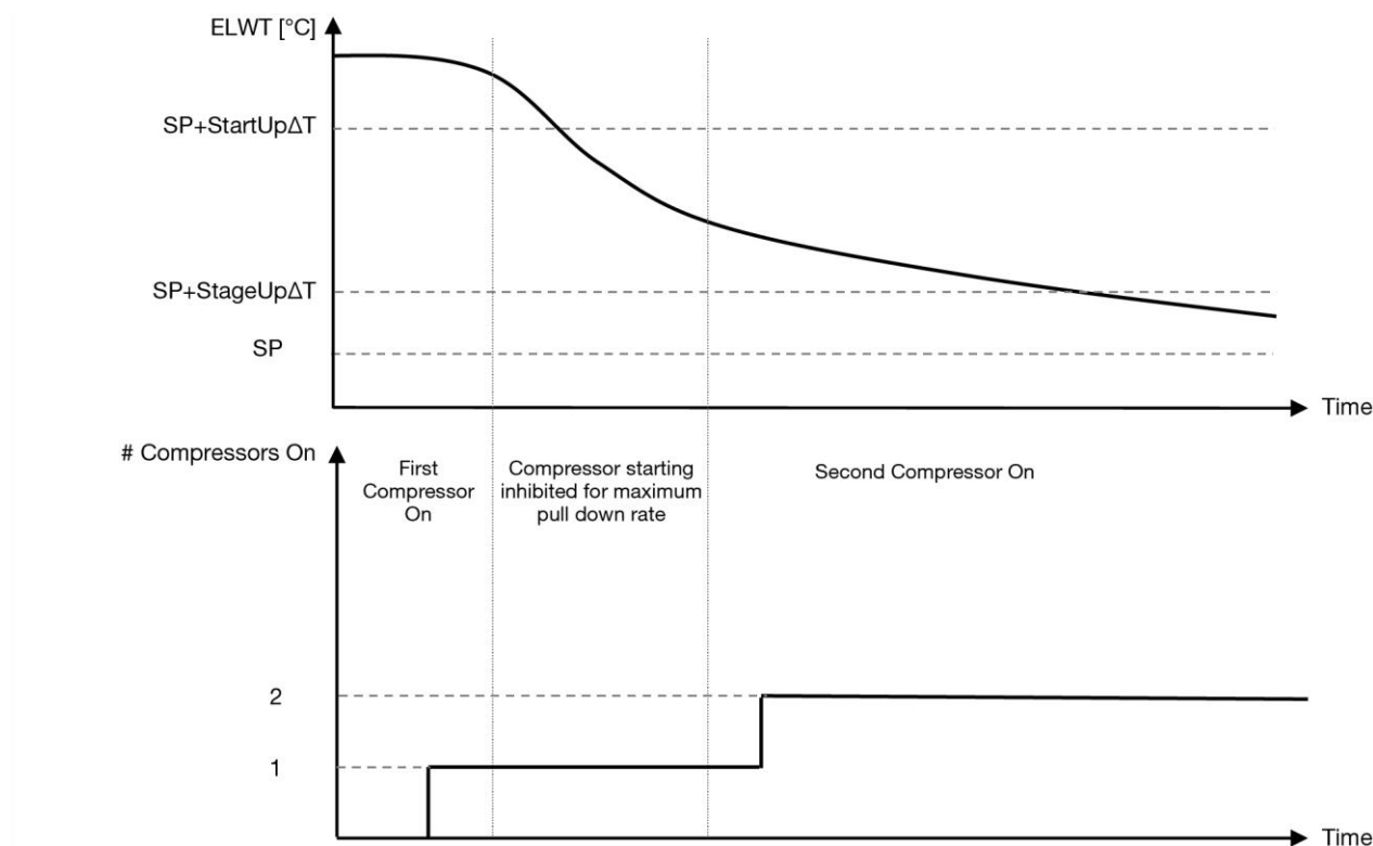
Diagram 1 – Kompressorns sekvens för uppstart - Kylläge
