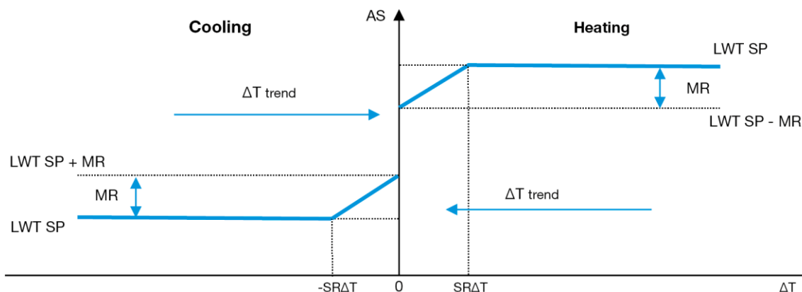
Grafico 3- Evap \Delta T vs Setpoint attivo - Modalità raffreddamento (sinistra) / Modalità riscaldamento (destra)
