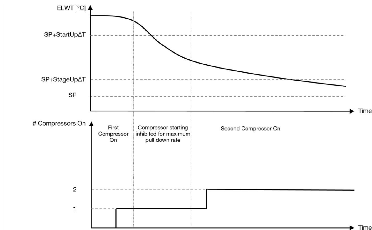
Grafikon 1- A kompresszorok indítási sorrendje - Hűvös üzemmód
