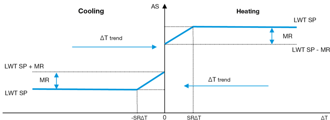
Grafikon 3 - Evap \Delta T vs. aktív beállítási pont - hűtési üzemmód (balra)/fűtési üzemmód (jobbra)
