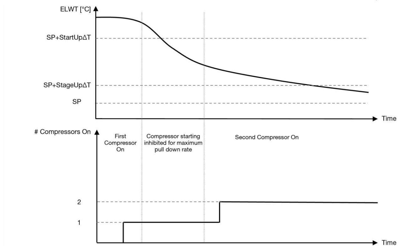
Grafik 1 - Startsequenz der Verdichter - Kühlbetrieb
