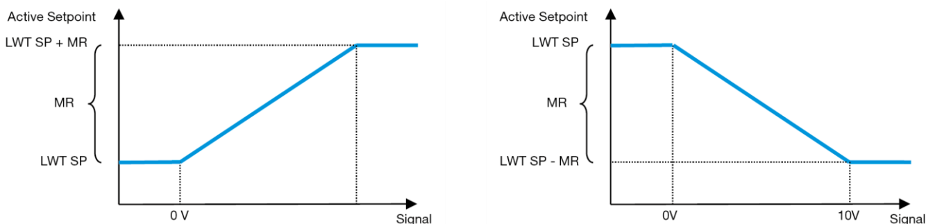
Graphique 2 - Signal externe 0-10 V vs Point de consigne actif - Mode refroidissement (gauche) / Mode chauffage (droite)
