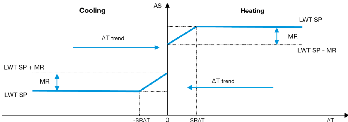
Graphique 3 - Evap \Delta T vs Active Setpoint - mode refroidissement (gauche)/mode chauffage (droit)
