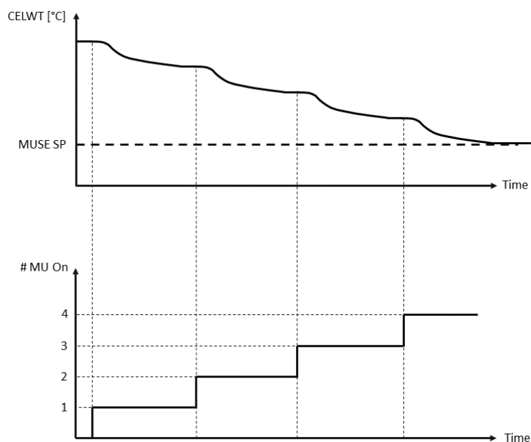
Graphique 4 - Séquence de démarrage des unités modulaires - Mode froid
