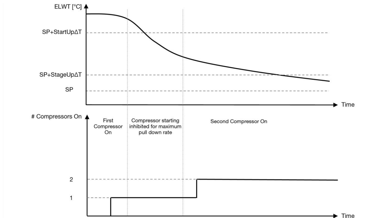
Graphique 1- Séquence de démarrage des compresseurs - Mode froid
