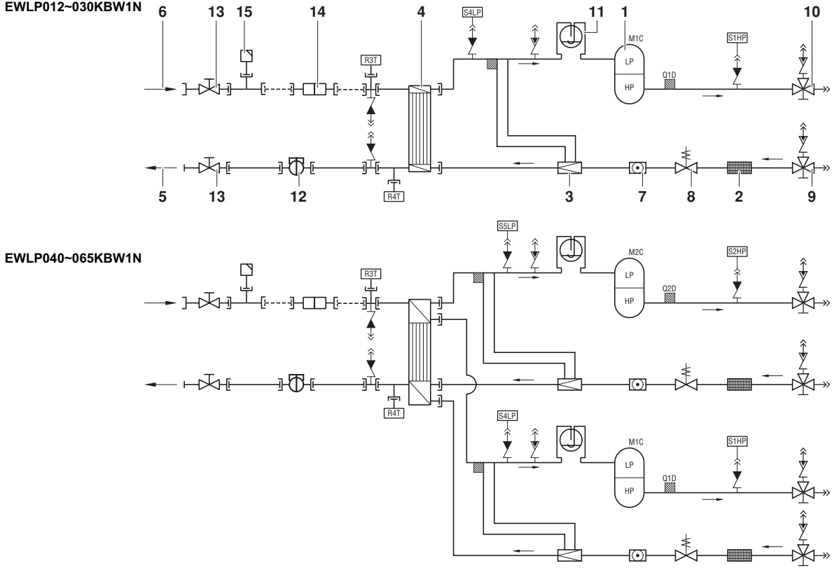
Şekil - İşlevsel şema
