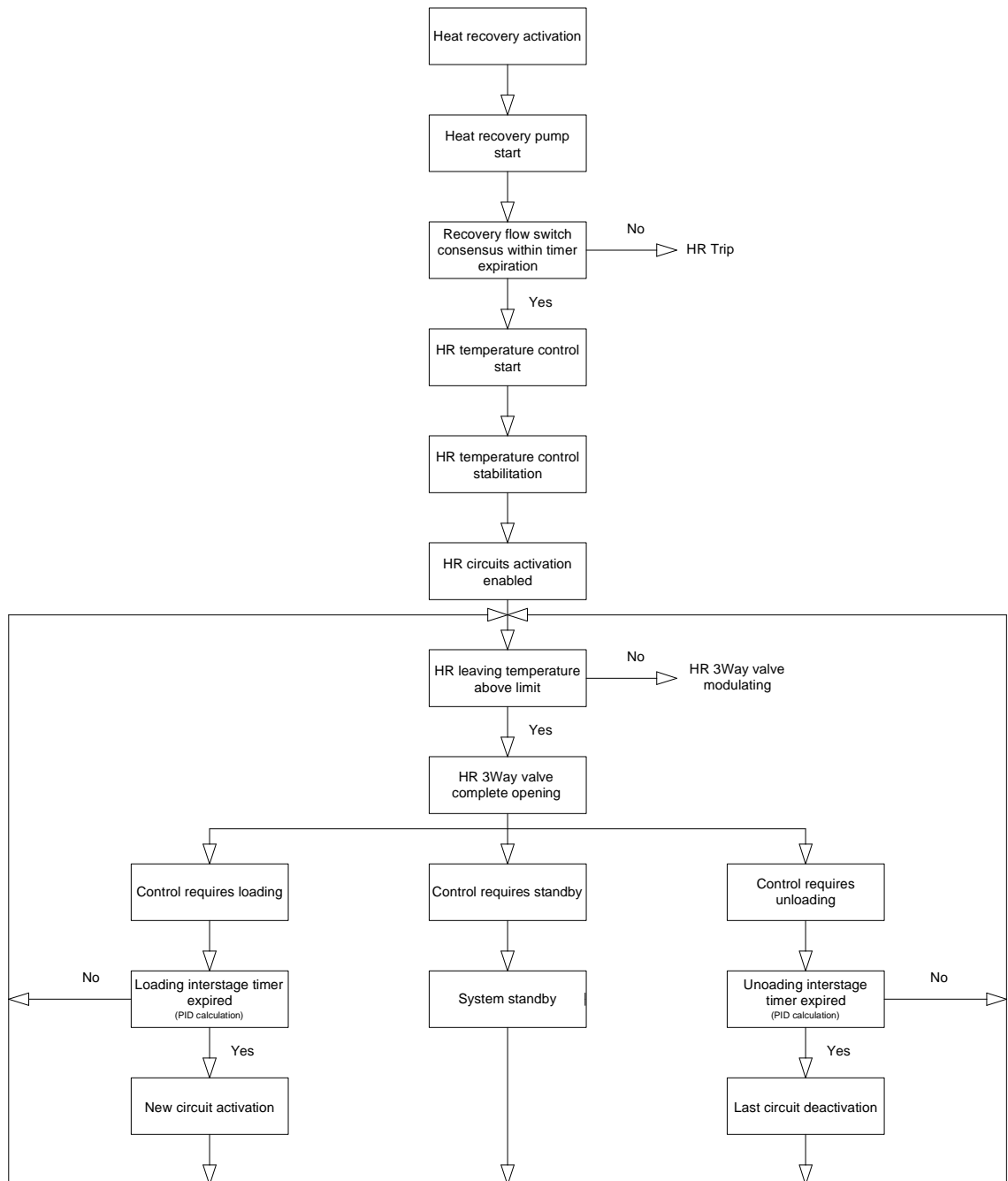
Afbeelding 19 – Opstartsequentie warmteterugwinning
