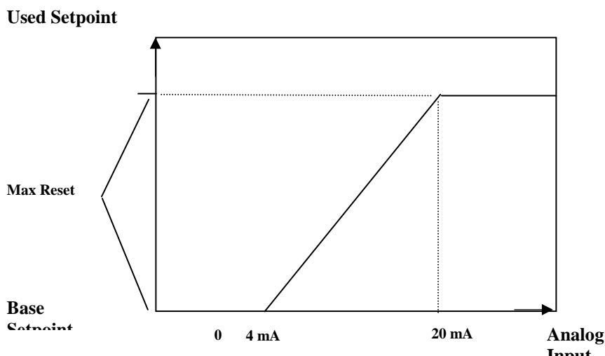
Afbeelding 8 – Tijdelijke opheffing instelpunt met 4-20mA-sigitaal
