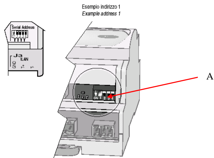
Afbeelding 6 – pCO e detail: schakelaars
