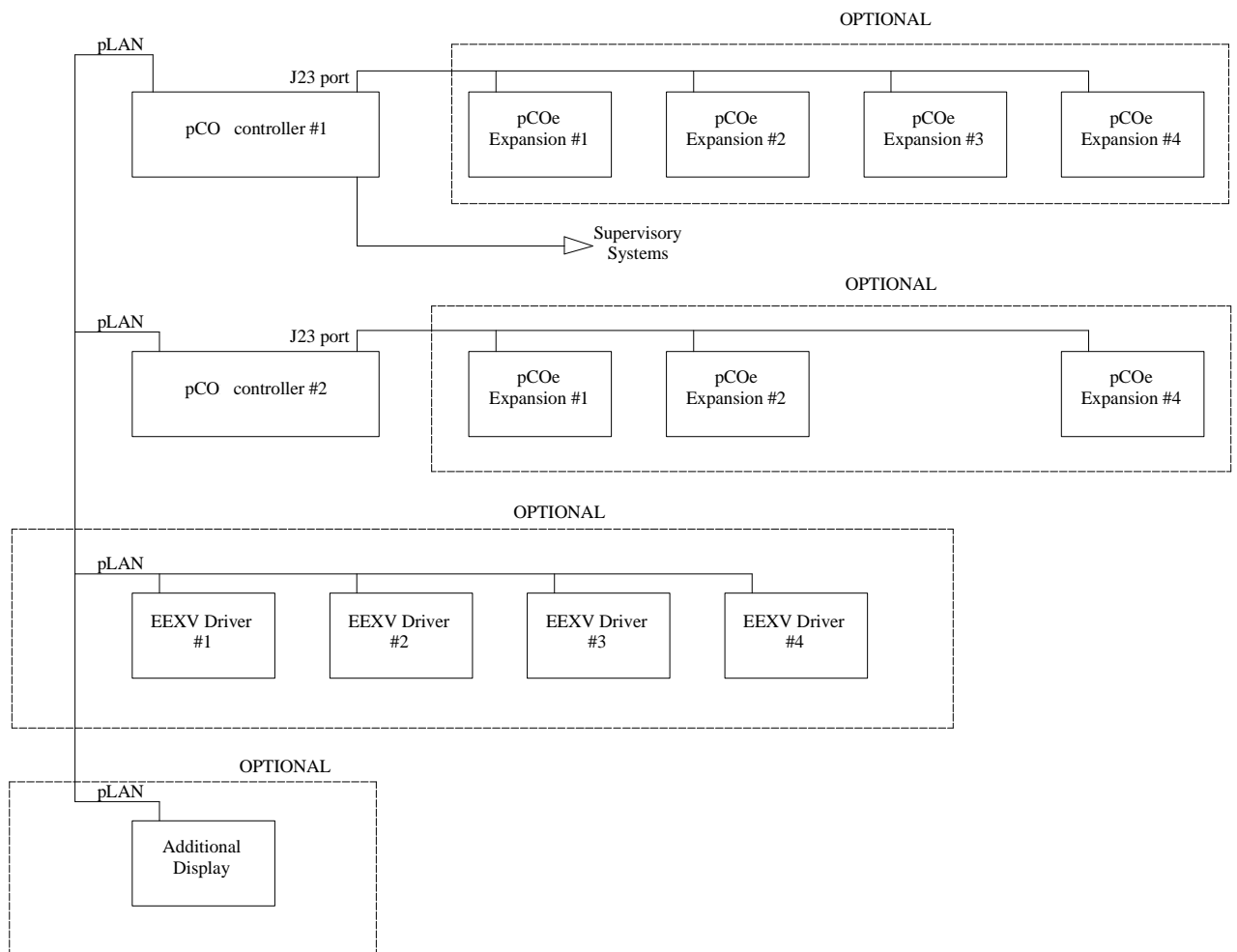
Afbeelding 1 – Lay-out van controller
