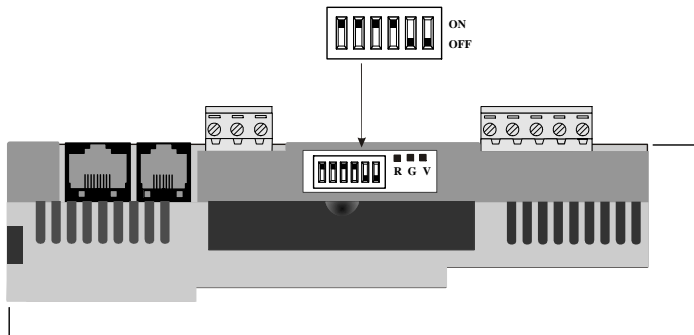
Microschakelaars adressering
