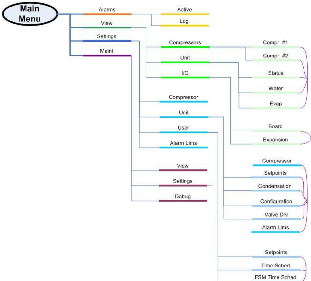
Fig 24 – Albero delle maschere
