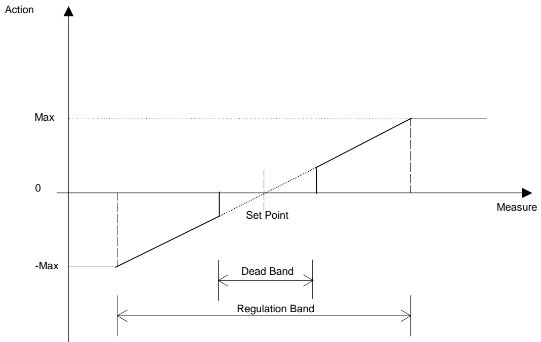
Fig. 12.– Azione proporzionale del controllore PD
