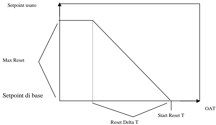
Fig. 9 – Reset del setpoint da temperatura esterna
