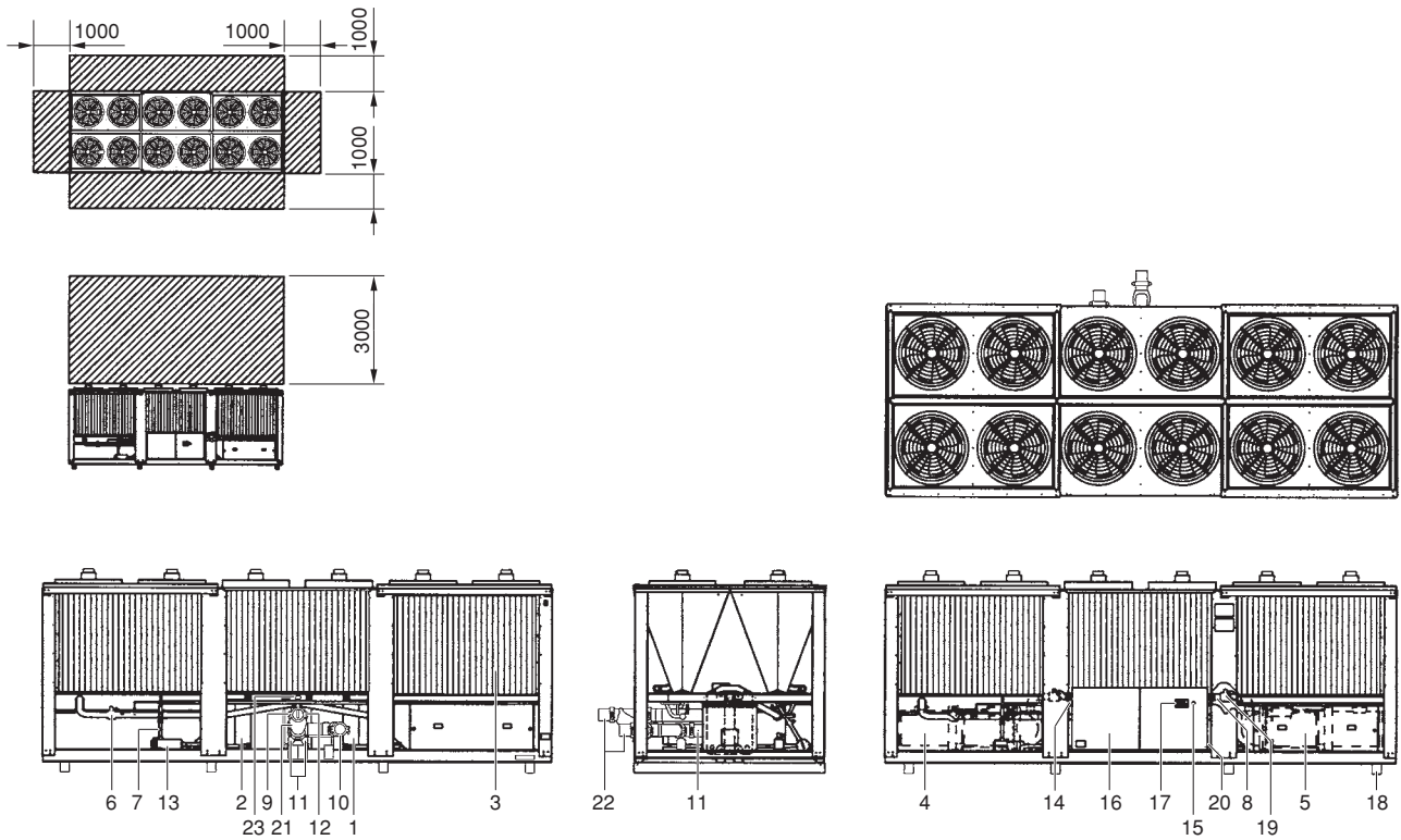
Figur - Hovedkomponenter
