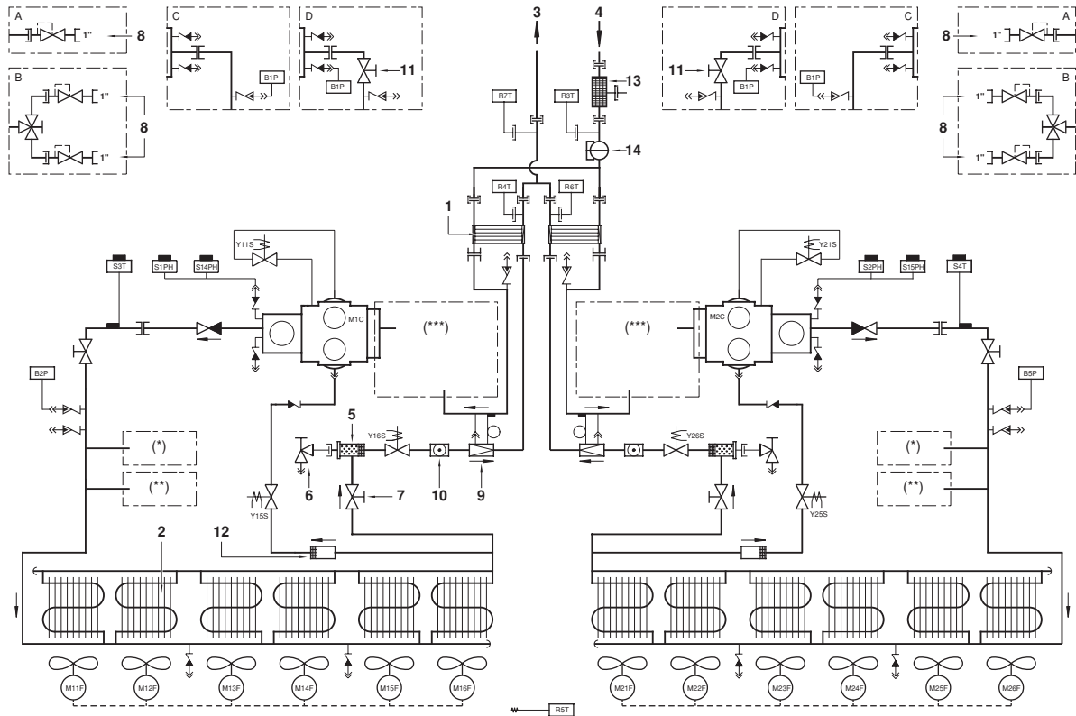
Figure - Schéma fonctionnel
