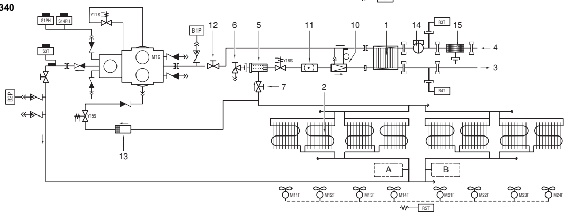
Obrázok - Funkčná schéma
