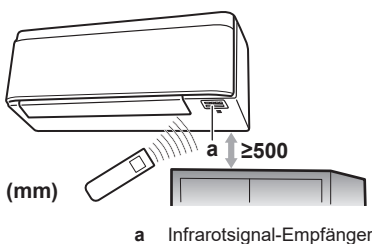
a Infrarotsignal-Empfänger
