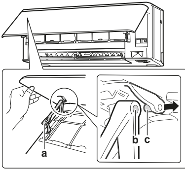
a Kol b Mil yuvası c Mil
