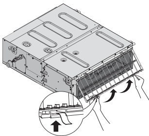
sucção traseira
