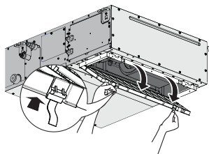
sucção inferior
