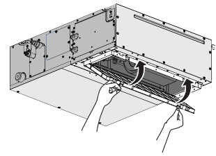
sucção inferior
