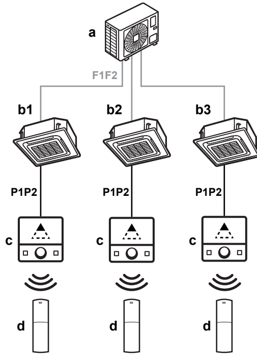
a الوحدة الخارجية المشتركة b الوحدة الداخلية c وحدة تحكم عن بُعد رئيسية d مستشعر الباب/النافذة (WLDW)
