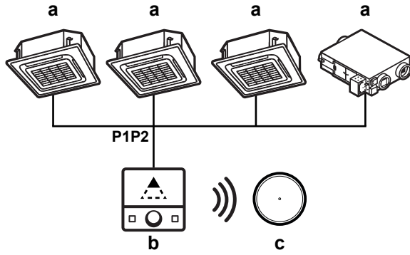
a الوحدات في المجموعة b وحدة تحكم عن بُعد رئيسية c مستشعر درجة الحرارة/الرطوبة (WLTRH)
