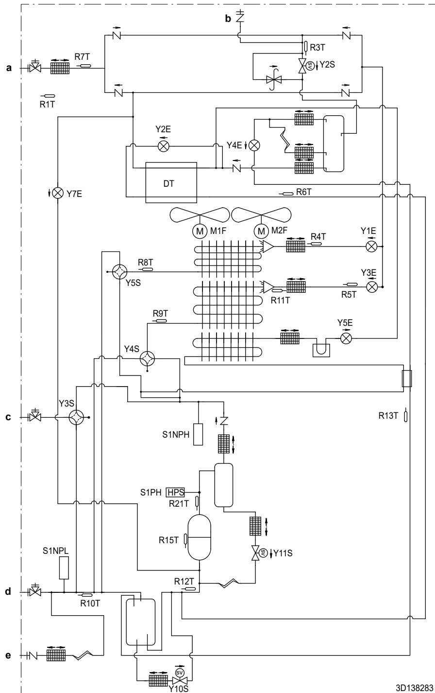
Rördragningschema: 14~20 HP
