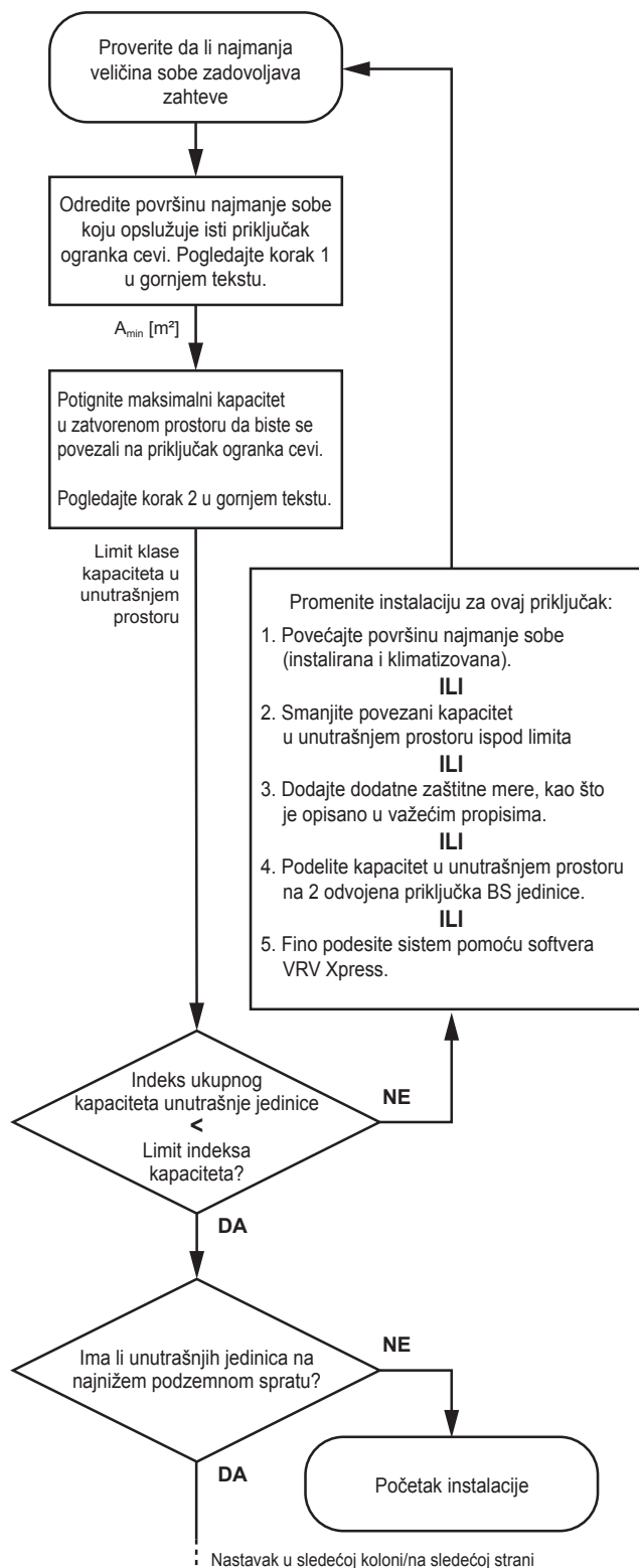
Dijagram toka (za OBA priključka ogranka cevi BS jedinice)
