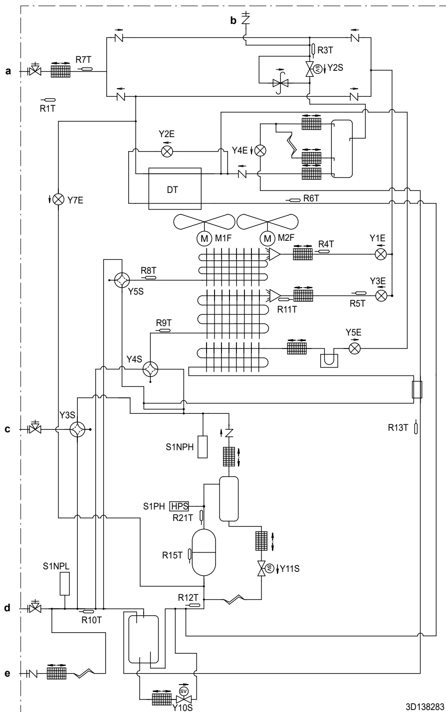
Schema tubulaturii: 14~20 HP
