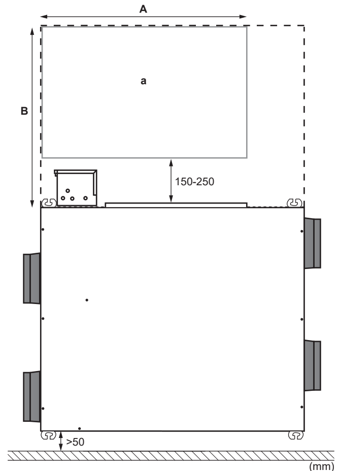
a Platz für Wartungsarbeiten
