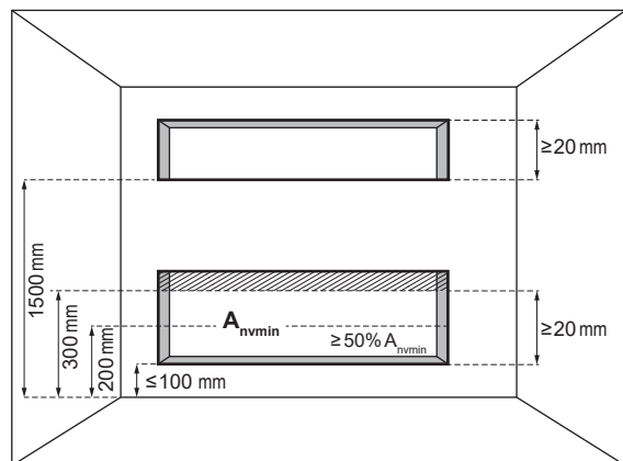
A_{nmin} Minimálna prirodzená plocha vetrania
