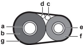
a Cijev za plin b Izolacija cijevi za plin c Kabel za međuvezu d Vanjsko ožičenje (ako je primjenjivo) e Cijev za tekućinu f Izolacija cijevi za tekućinu g Završna traka
