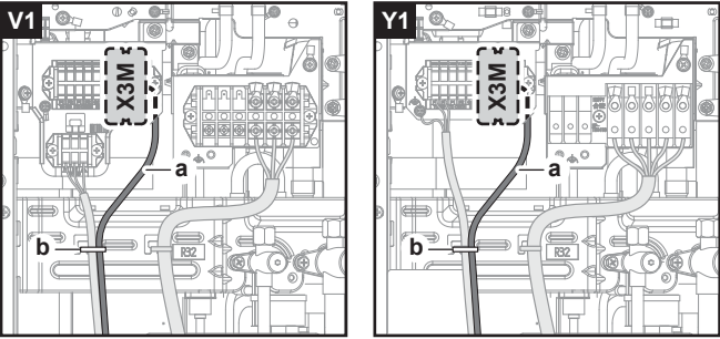
a Kabel izborne sklopke hlađenje/grijanje b Kabelska vezica
