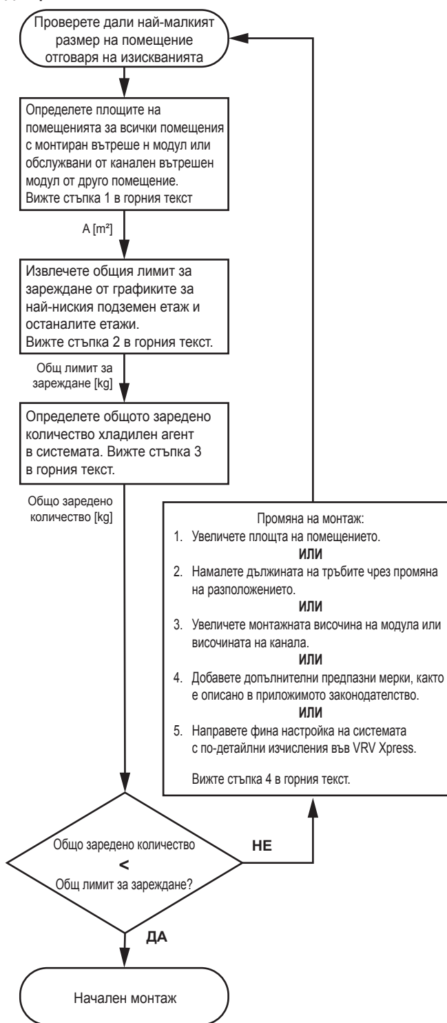
Диаграма на потока
