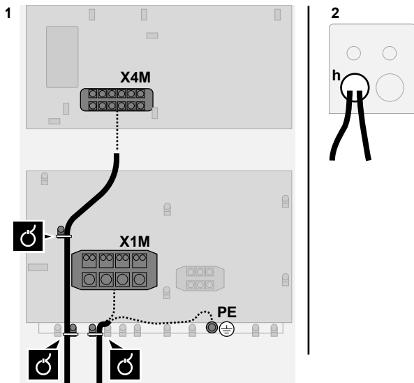
h Bedradingsinlaat (uitbrekopening) voor hoogspanning. Zie "14.3 Richtlijnen bij het uitslaan van de uitbrekopeningen" [p. 36].
