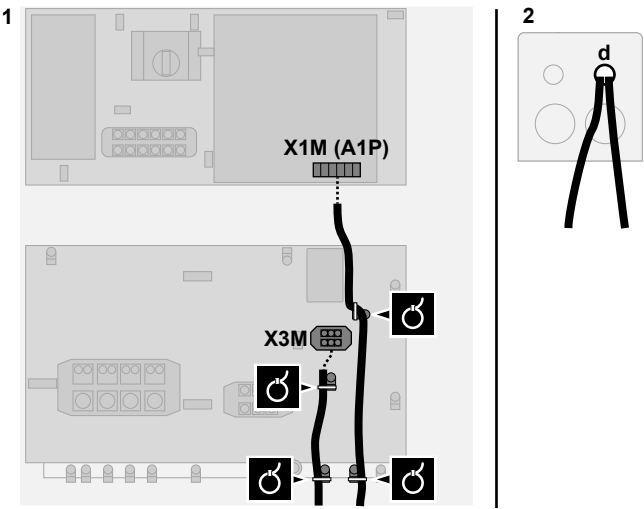
d Bedradingsinlaat (uitbreekopening) voor laagspanning. Zie "14.3 Richtlijnen bij het uitslaan van de uitbreekopeningen" [p. 36].
