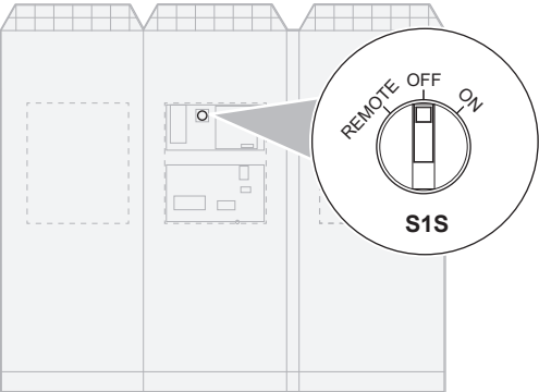
S1S In de fabriek geïnstalleerde bedrijfsschakelaar: OFF: Unit werking UIT ON: Unit werking AAN Remote: Unit gestuurd (AAN/UIT) met schakelaar bediening op afstand
