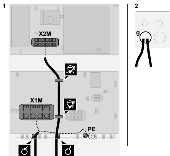
g Bedradingsinlaat (uitbreekopening) voor hoogspanning. Zie "14.3 Richtlijnen bij het uitslaan van de uitbreekopeningen" [p. 36].
