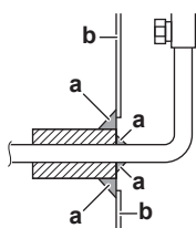
a Μονωτικό υλικό b Πρόσωση
