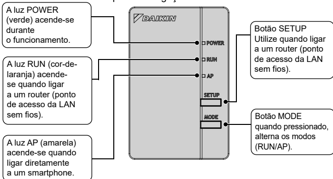
Adaptador de ligação da LAN sem fios
