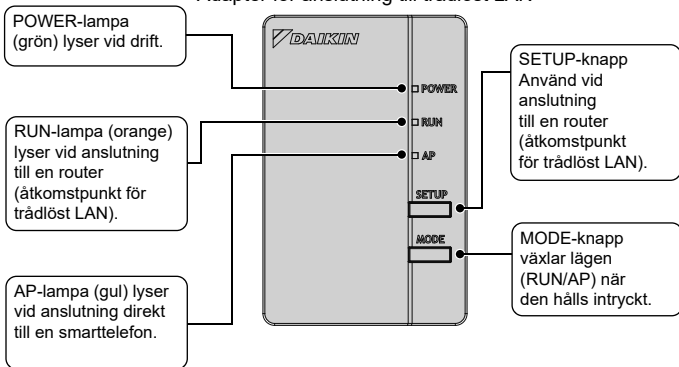
Adapter för anslutning till trådlöst LAN
