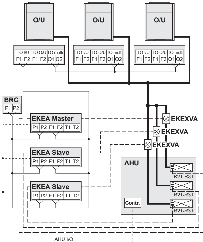
Zgled kombiniranega sistemskega tokokroga hladiva:
