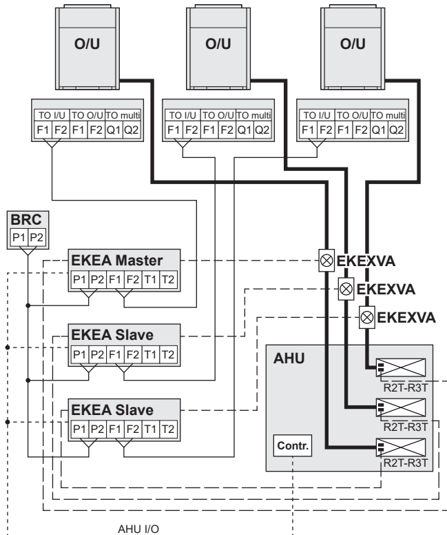
Zgled ločenega sistemskega tokokroga hladiva:
