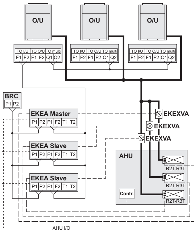
Exemplo de sistema de circuito de refrigerante combinado:
