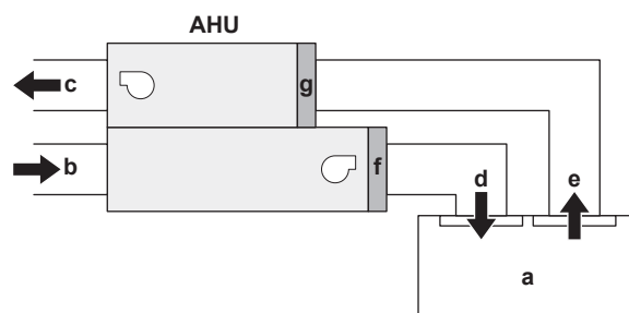
AHU Luchtbehandelingsunit
