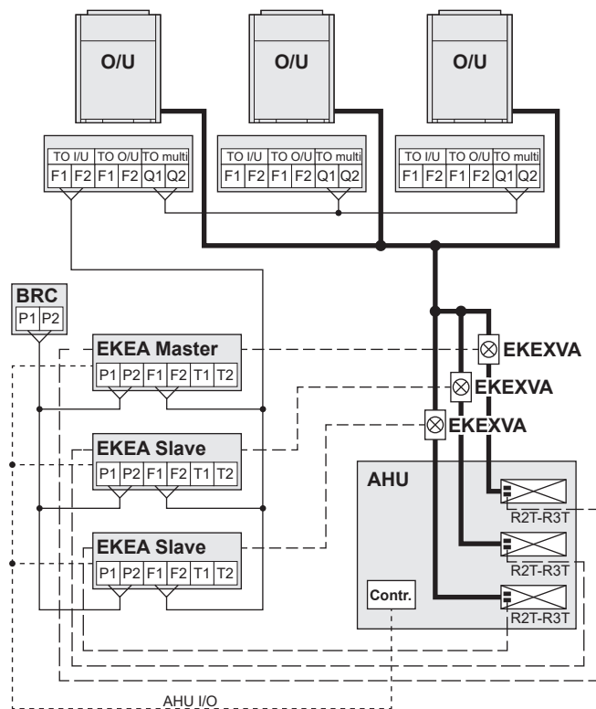
Παράδειγμα συστήματος συνδυασμένου κυκλώματος ψυκτικού:
