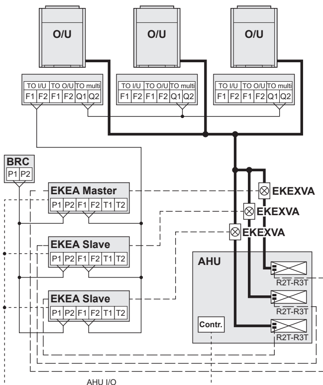
Eksempel system med kombineret kølemiddelkreds:
