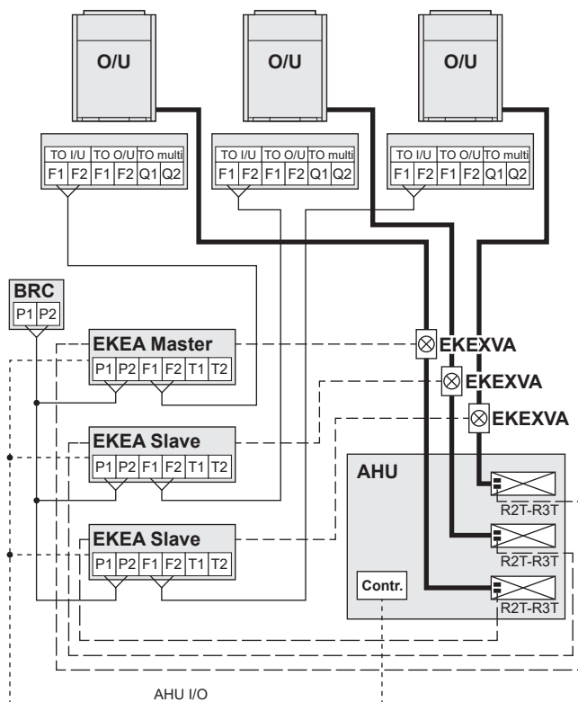
Eksempel system med separat kølemiddelkreds:
