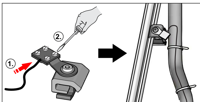
Bild 4-20 Arbeitsschritte 1+2
