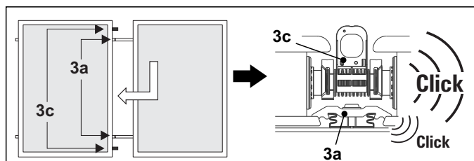
Bild 4-9 Arbeitsschritt 6 bei 2 und mehr Kollektoren
