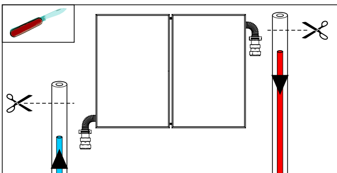
Bild 4-17 Arbeitsschritt 5
