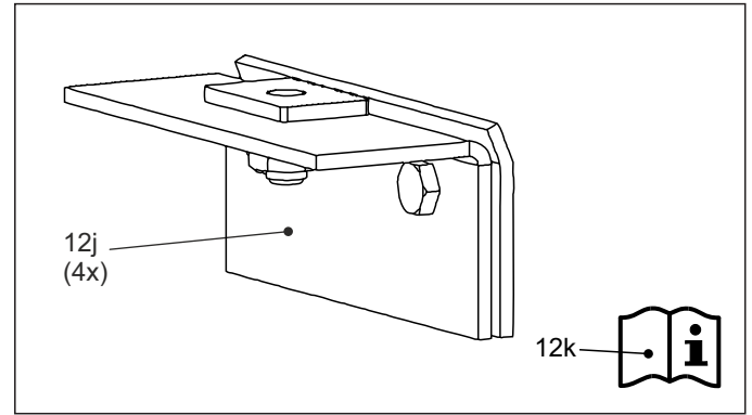
Bild 3-14 FIX BD
