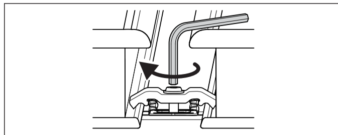
Bild 4-10 Arbeitsschritt 7
