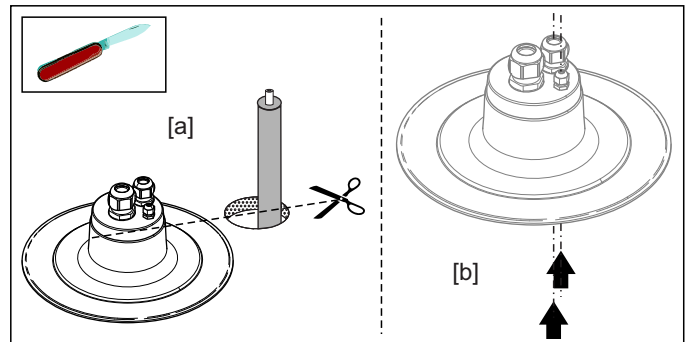
Bild 4-4 Arbeitsschritte 5a und 5b
