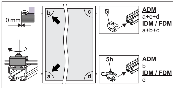
Bild 4-7 Arbeitsschritt 4
