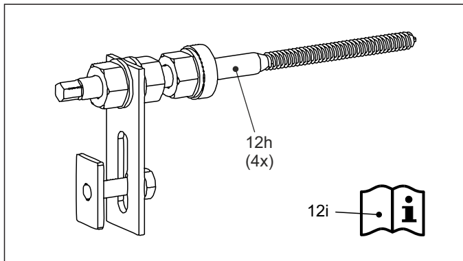
Bild 3-13 FIX WD
