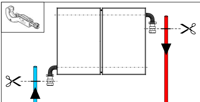
Bild 4-16 Arbeitsschritt 4
