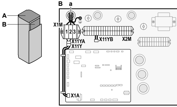
a Ara bağlantı kablosu (=ana güç kaynağı)
