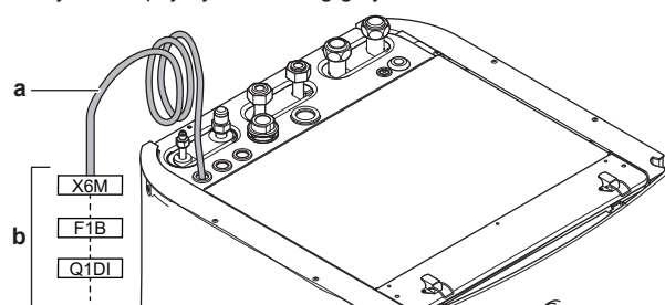
a Fabrički montiran kabl povezan sa kontaktom rezervnog grejača, unutar razvodne kutije (K5M)
