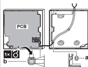
4A Підключення ззаду
