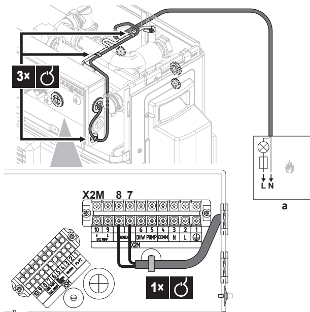
a Бівалентний сигнал для стороннього газового котла
