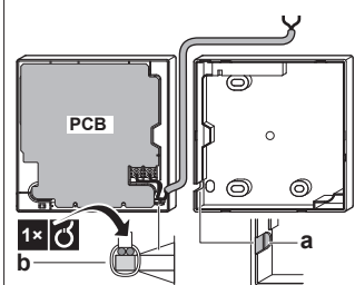
4B Підключення зліва
