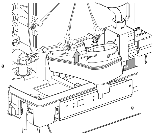
а Основний піддон
