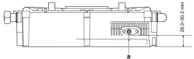
a Зазор між електродами (±4,5 мм)
