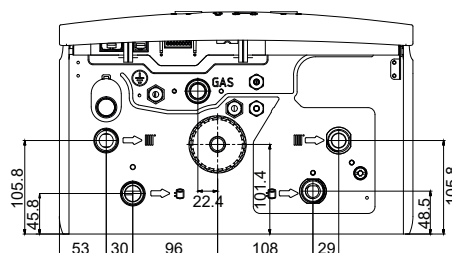
Pohľad na modely D2TND012A4AB, D2TND018A4AB a D2TND024A4AB zospodu
