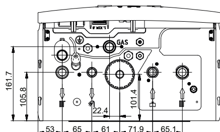
Pohľad na model D2CND024A1AB zospodu
