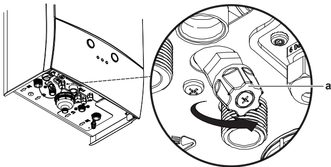
a Plniaci ventil
