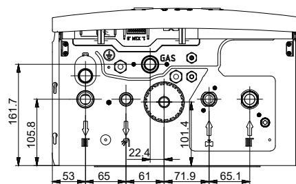
Pohľad na modely D2TND012A4AB, D2TND018A4AB a D2TND024A4AB zospodu
